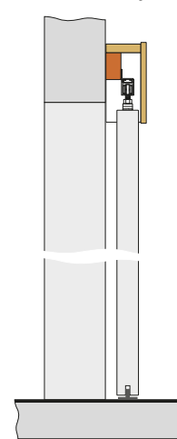
System naścienny zamontowany bez zabudowy
