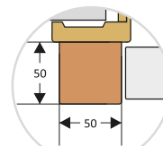
listwa odbojowa zamontowana na ościeżnicy
