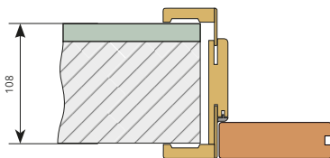
ościeżnica B (88-108 mm) grubość muru 110 mm opaska kątowa rozsunięta w zakresie 0-20 mm
