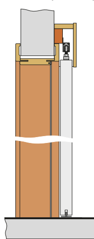
System naścienny zamontowany z zabudową tunelową
