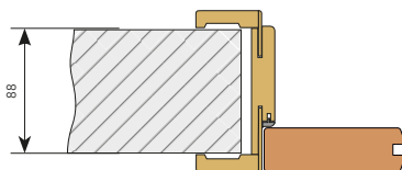
ościeżnica B (88-108 mm) grubość muru 90 mm opaska kątowa wsunięta
